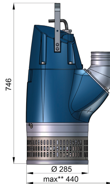
Warman SJX-5-HH-50Hz
